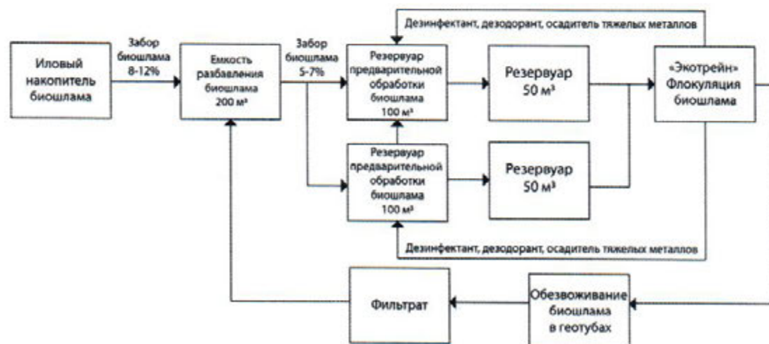
Рис. 2. Технологическая схема обработки биошлама из иловых карт
